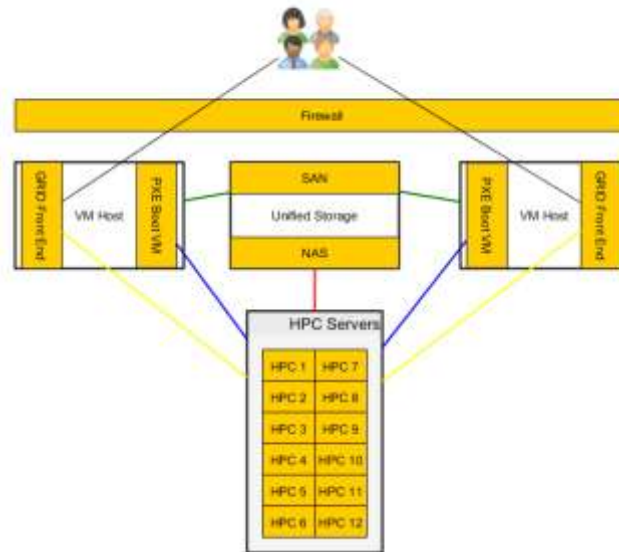
Εικόνα 2: Λογικό διάγραμμα της νέας υπηρεσίας του HPC
