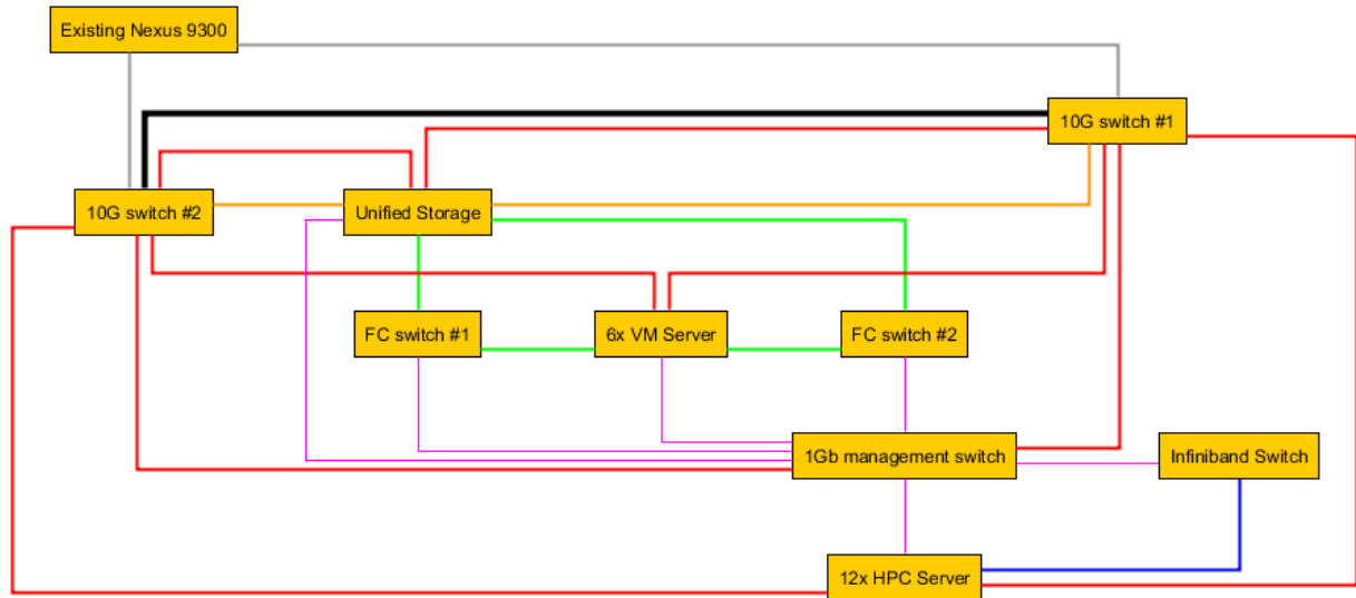
Εικόνα 1: Συνολική αποτύπωση της επιθυμητής συνδεσμολογίας: με μπλε χρώμα απεικονίζονται οι συνδέσεις Infiniband, με έντονο μαύρο χρώμα το stacking cable μεταξύ των δύο 10G switch, με πράσινο χρώμα οι συνδέσεις FC 16Gb/s, με κόκκινο χρώμα οι συνδέσεις 10G Ethernet SFP+ (twinax), με πορτοκαλί χρώμα οι συνδέσεις 10G iSCSI SFP+ (twinax), με γκρι χρώμα οι συνδέσεις 100Gb/s και με μώβ χρώμα οι συνδέσεις 1G Ethernet Base-T.
